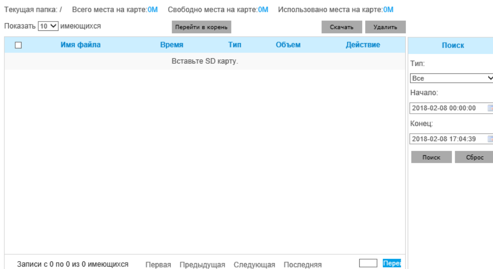
Рисунок 4-4-14 Просмотр SD-карты
