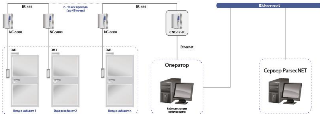
Рисунок 5. Место ЦКС в системе ParsecNET 3
