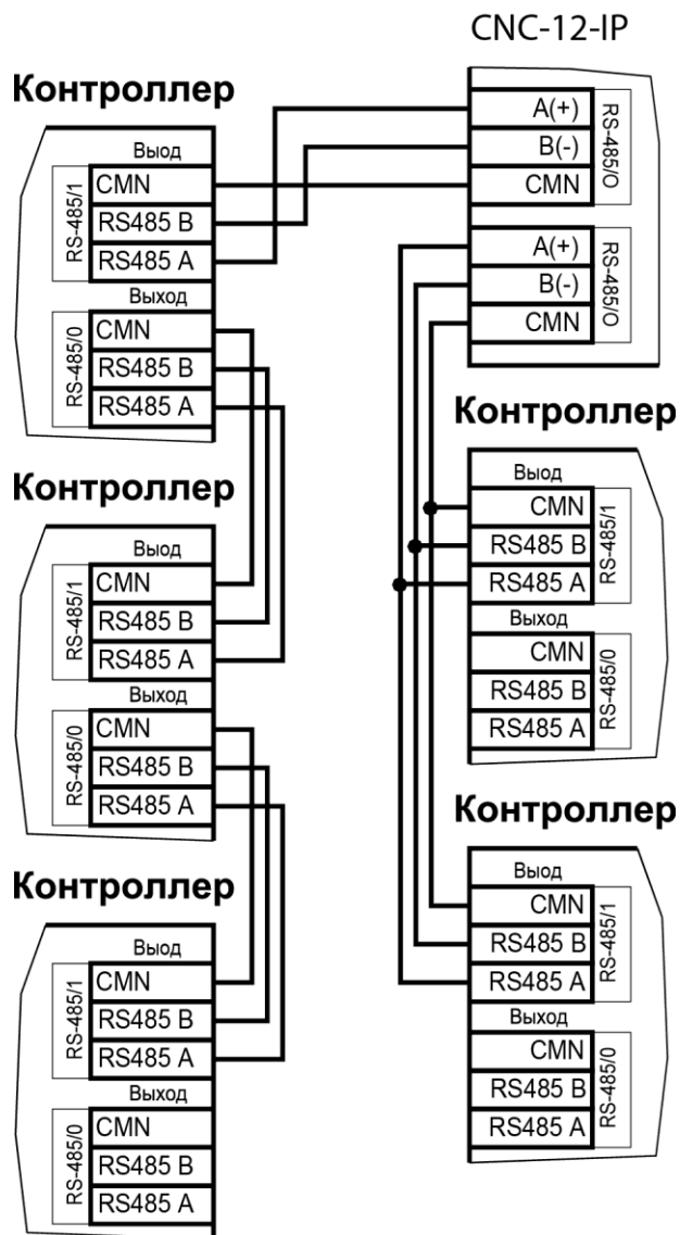
Рисунок 9. Подключение контроллеров по разным топологиям
