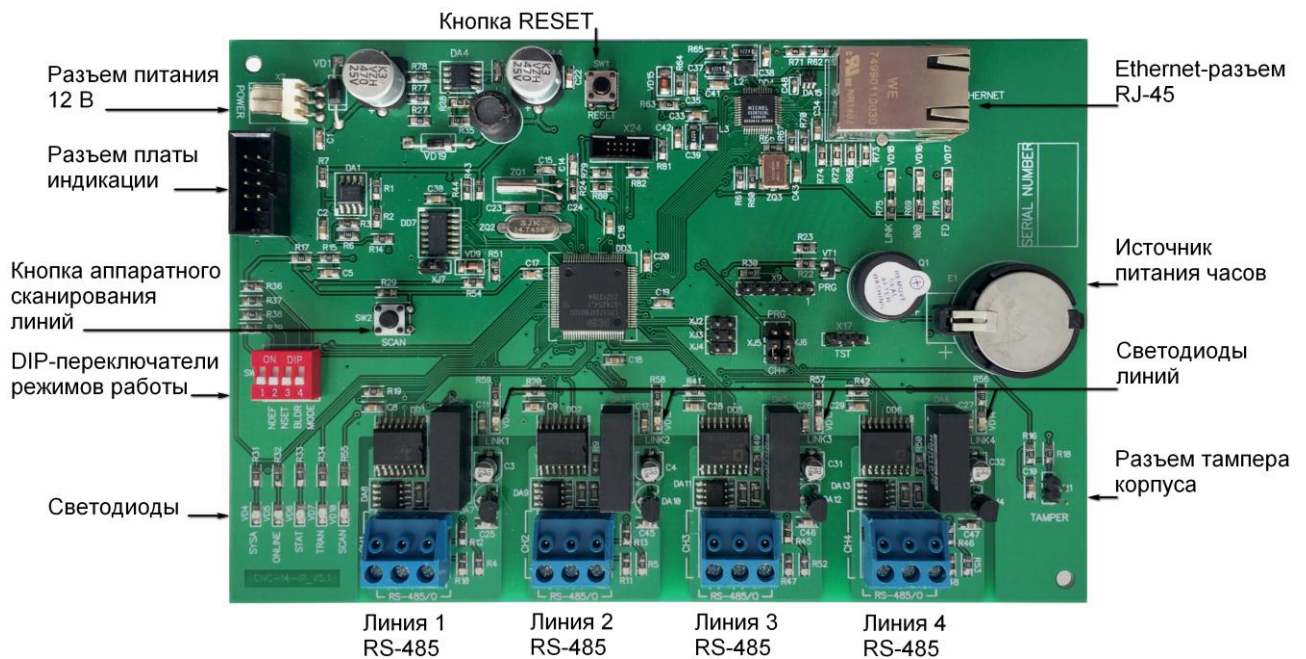
Рисунок 3. Плата CNC-14-IP
