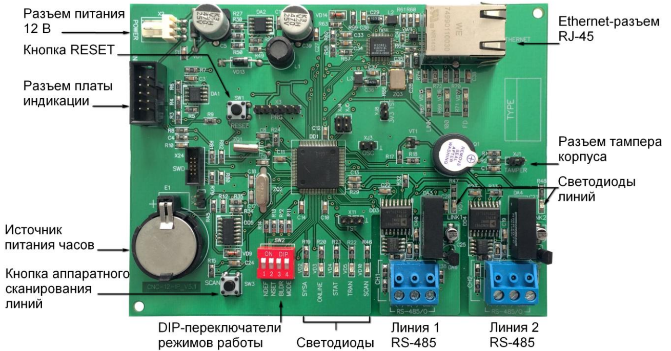
Рисунок 2. Плата CNC-12-IP
