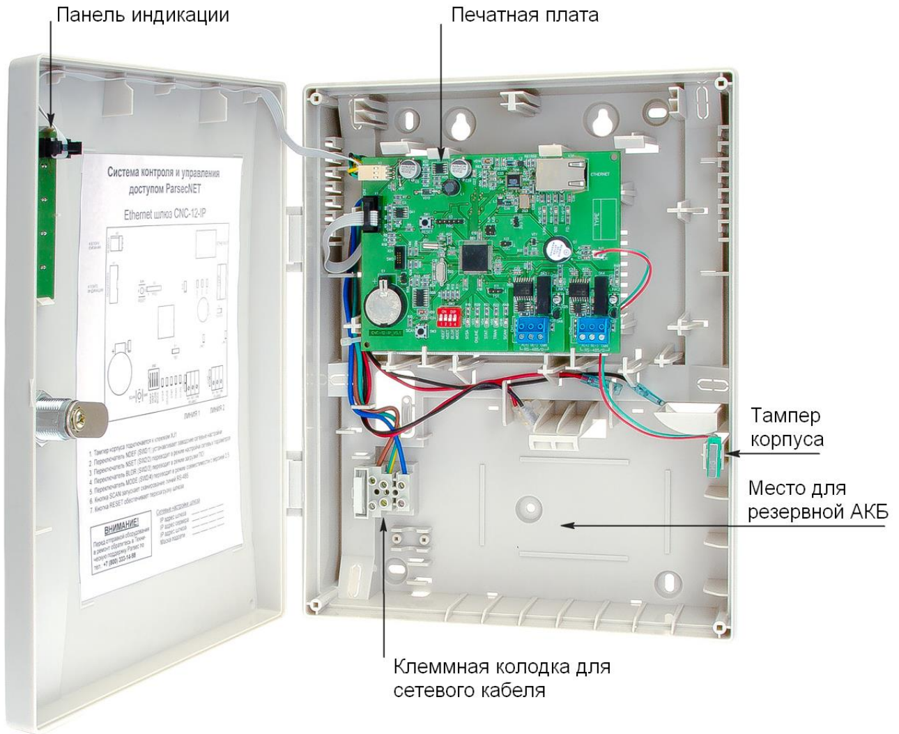
Рисунок 1. CNC-12-IP в открытом корпусе
