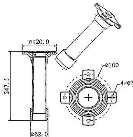
Рис. 5 Кронштейн крепления на горизонтальную поверхность.
