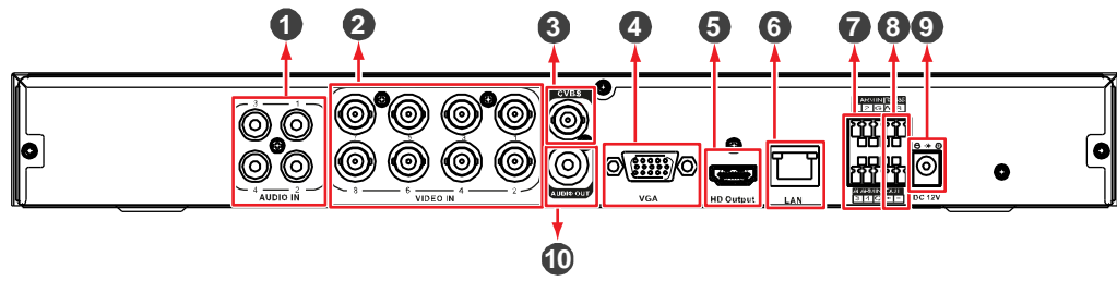
Рис. 2-2 Описание и разъемы задней панели 4-канального и 8-канального DVR
