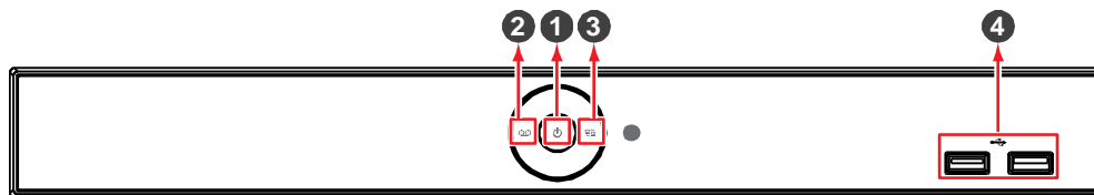
Рис. 2-1 Описание и разъемы передней панели
