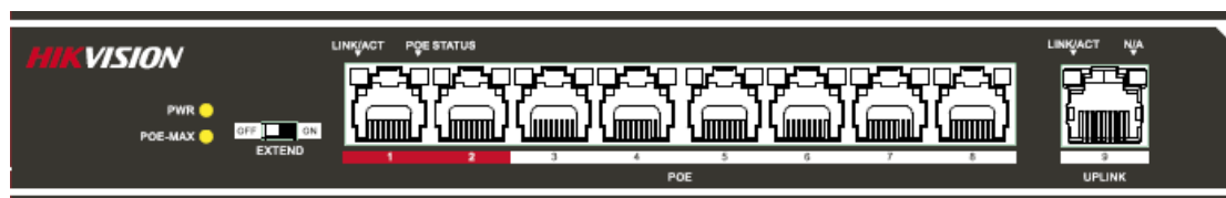
Рисунок 1.2 DS-3E0109P-E
