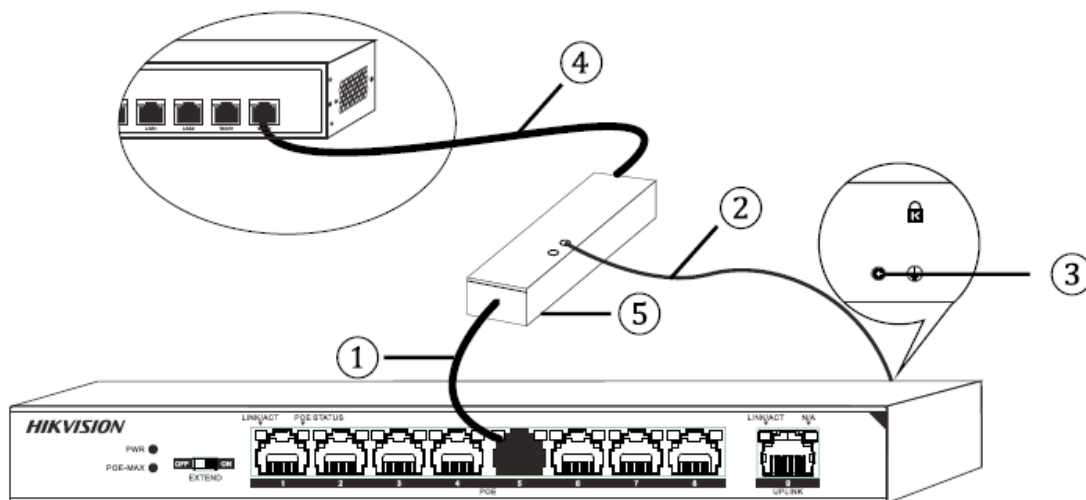
Рисунок 3.2 Подключение молниеотвода
