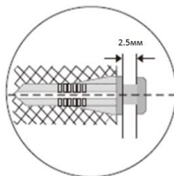
Рисунок 2.3 Установка шурупов
